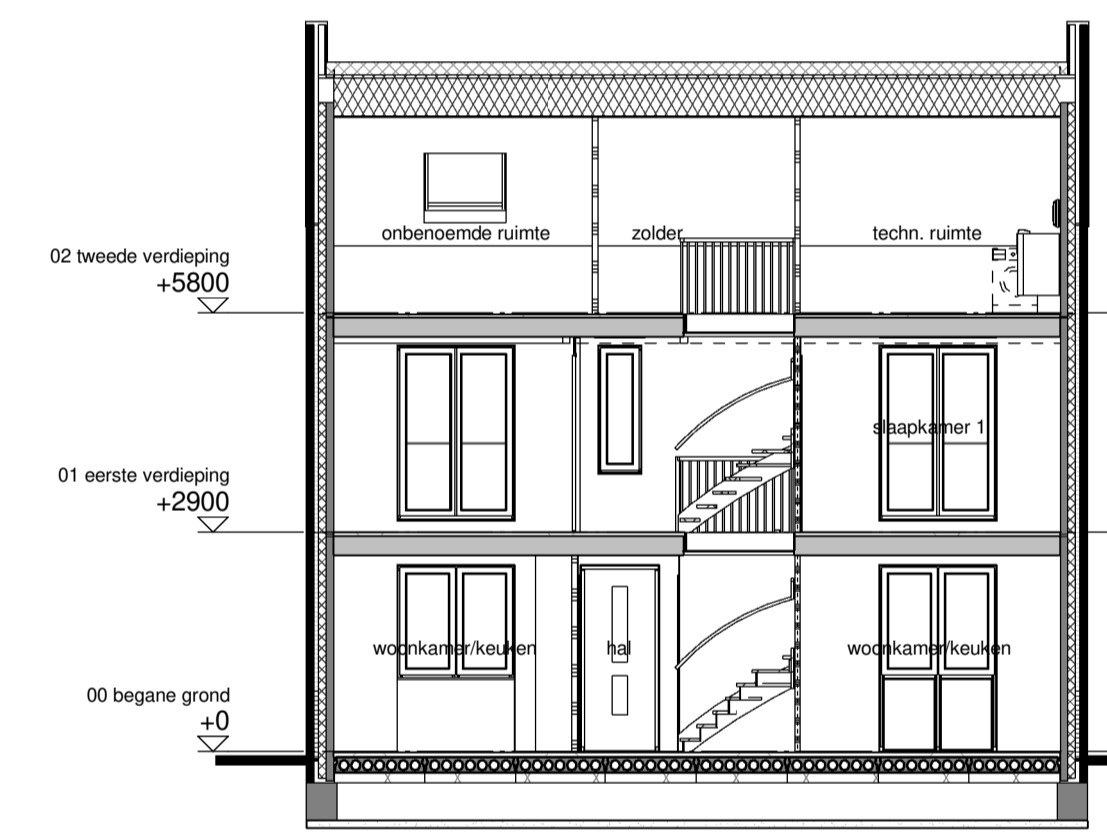
Doorsnede O schaal 1:100
