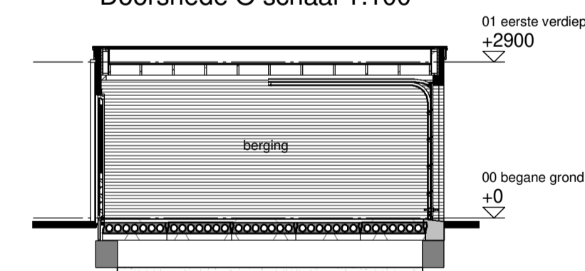
Doorsnede O schaal 1:100
