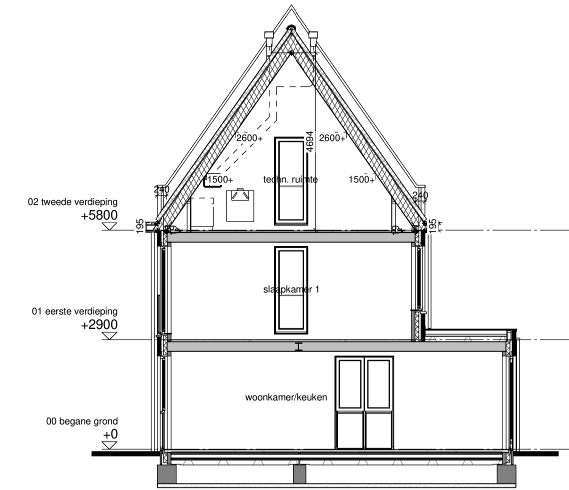
Doorsnede O2 schaal 1:100
