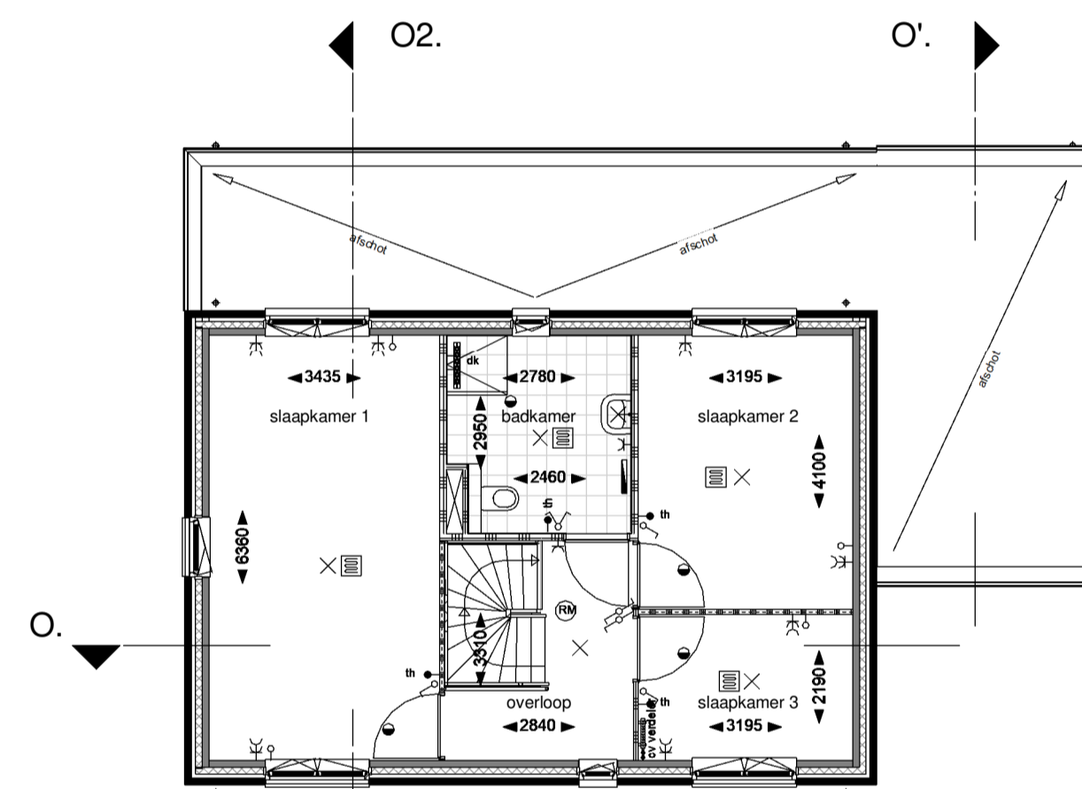
Eerste verdieping schaal 1:100
