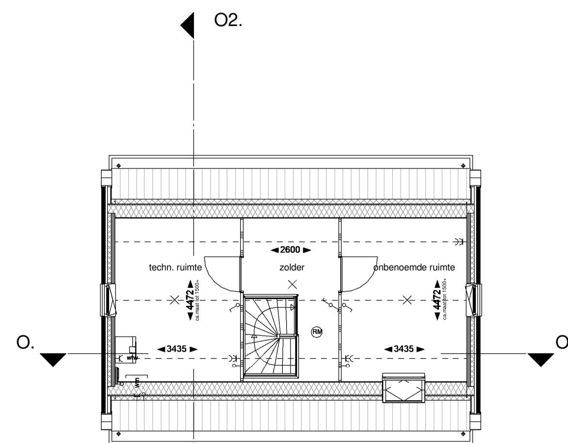
Tweede verdieping schaal 1:100
