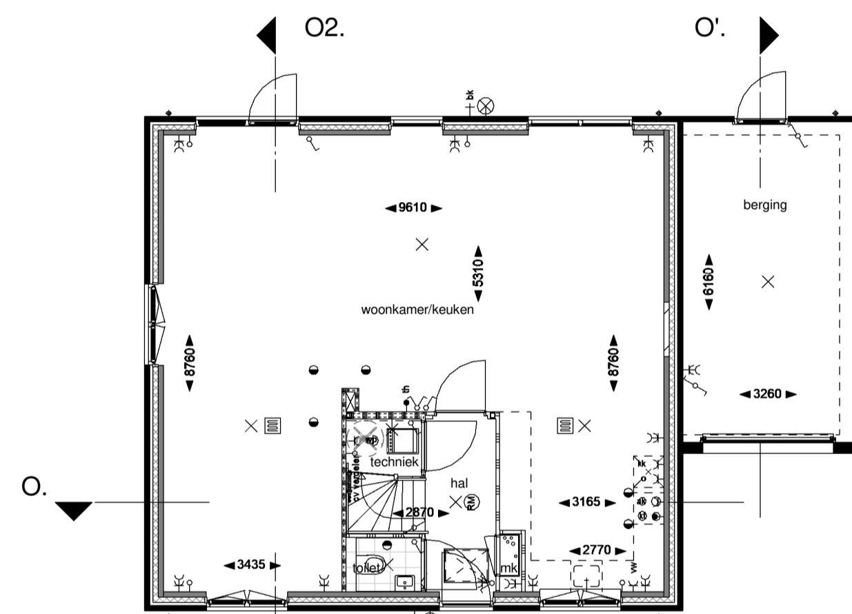
Begane grond schaal 1:100
