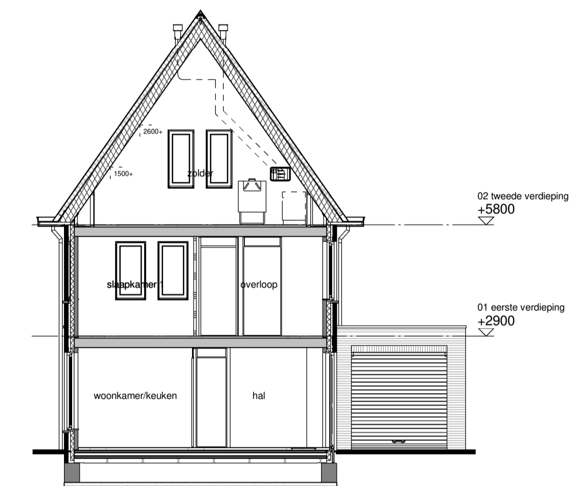
Doorsnede K2 schaal 1:100
