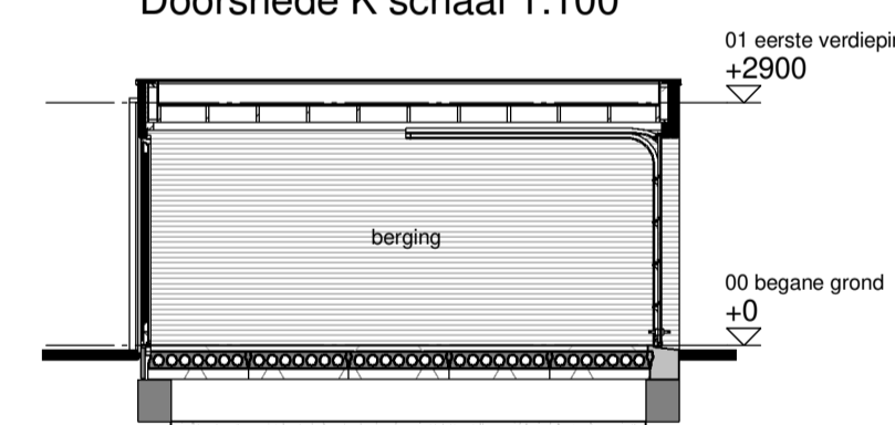
Doorsnede K schaal 1:100
