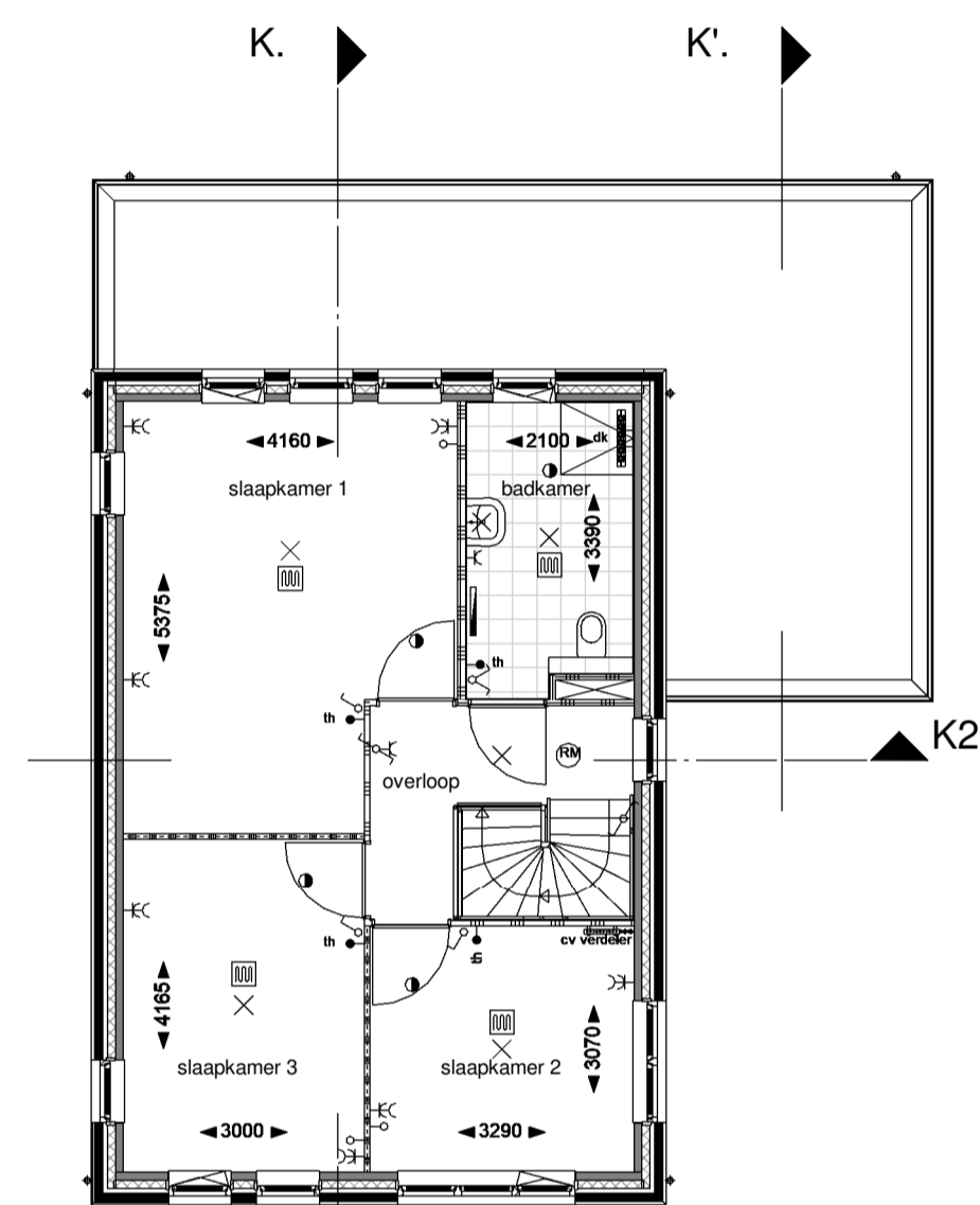
Eerste verdieping schaal 1:100
