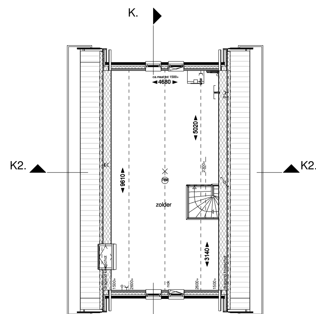
Tweede verdieping schaal 1:100
