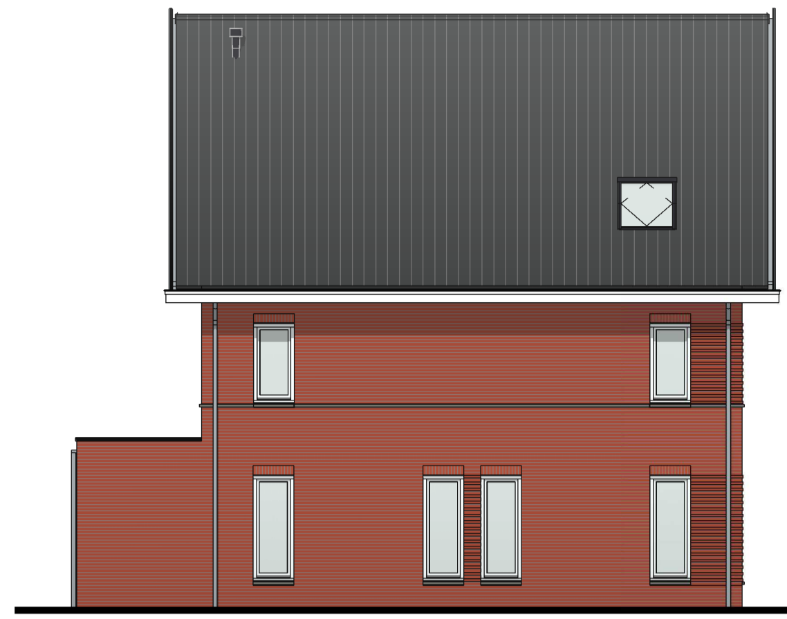
Linker zijgevel schaal 1:100
