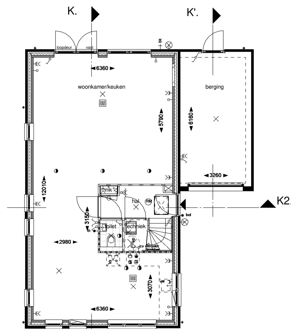
Begane grond schaal 1:100
