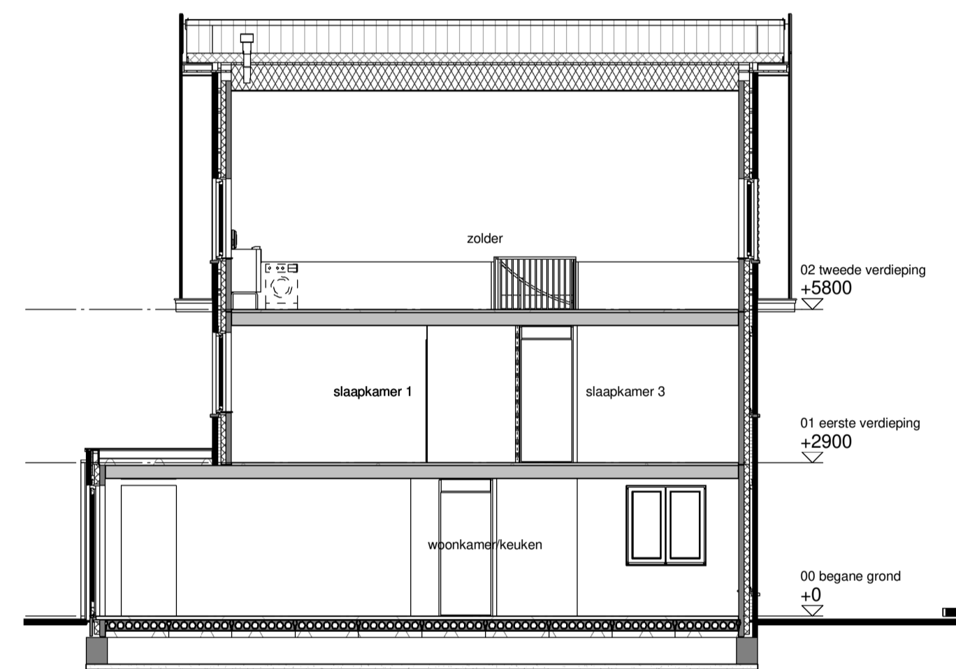
Doorsnede K schaal 1:100
