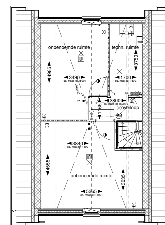
Tweede verdieping
