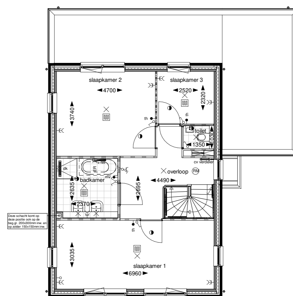
Eerste verdieping
