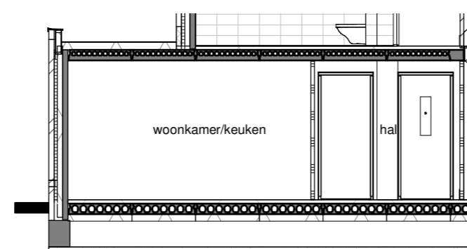
Doorsnede
