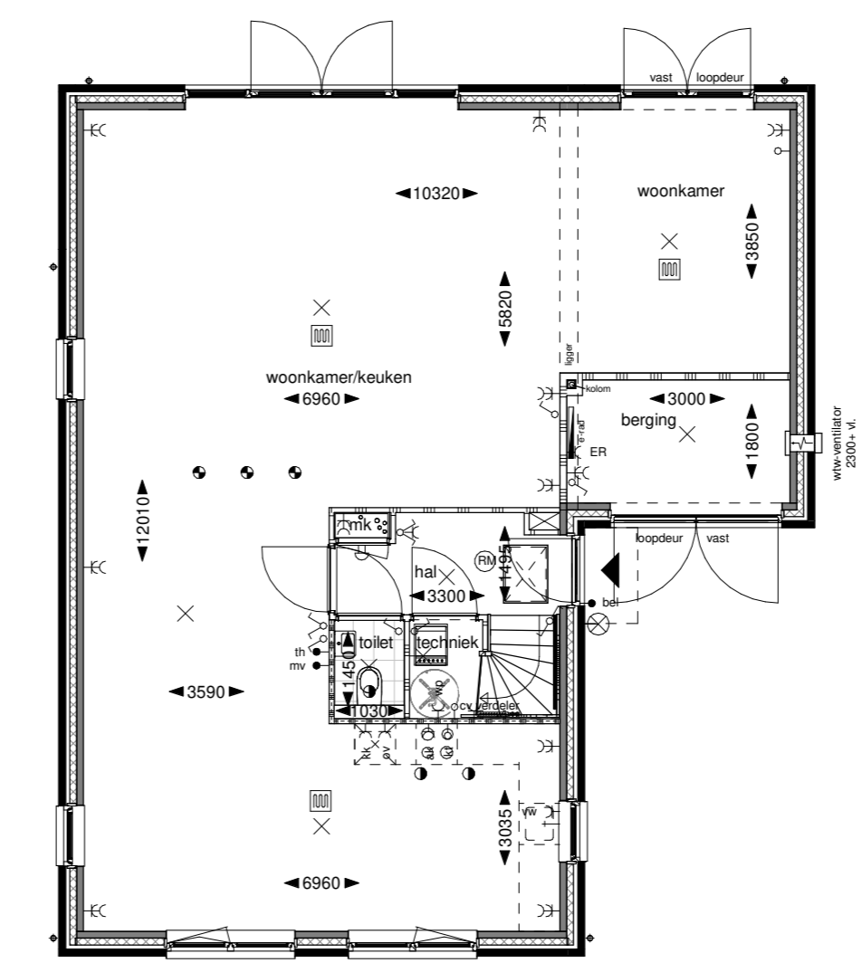
Begane grond
