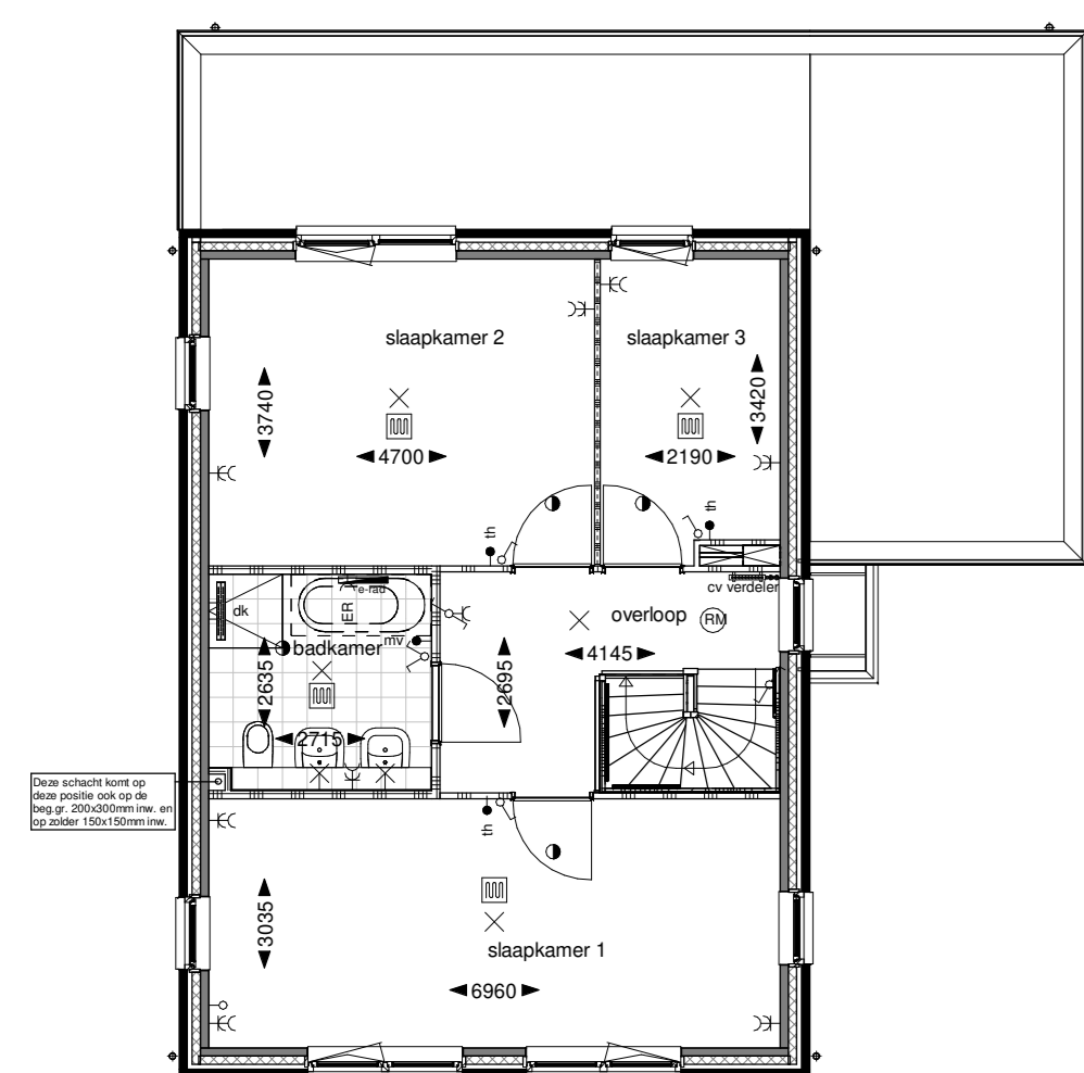
Eerste verdieping
