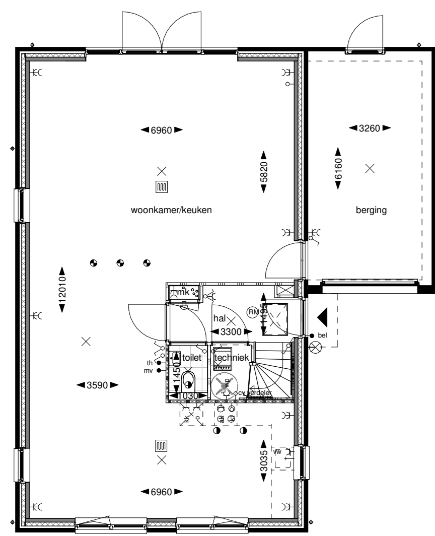
Begane grond
