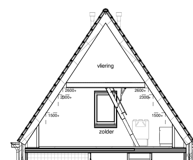
Doorsnede
