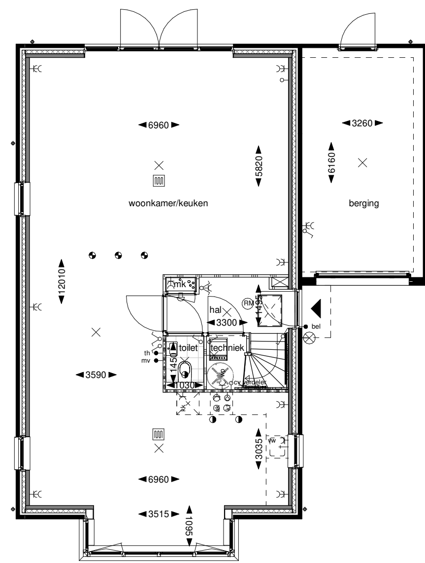
Begane grond
