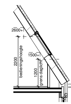
Doorsnede
