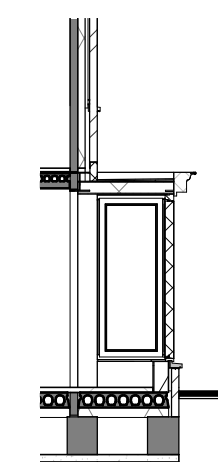
Doorsnede
