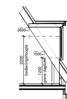
Doorsnede
