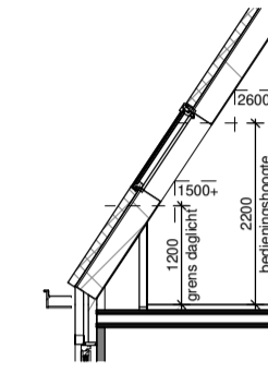
Doorsnede
