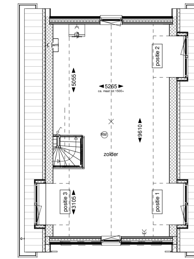
Tweede verdieping
