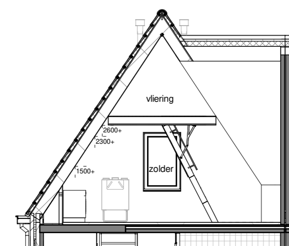
Doorsnede
