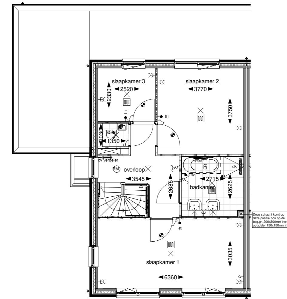
Eerste verdieping
