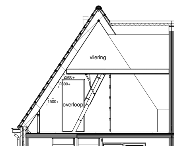
Doorsnede
