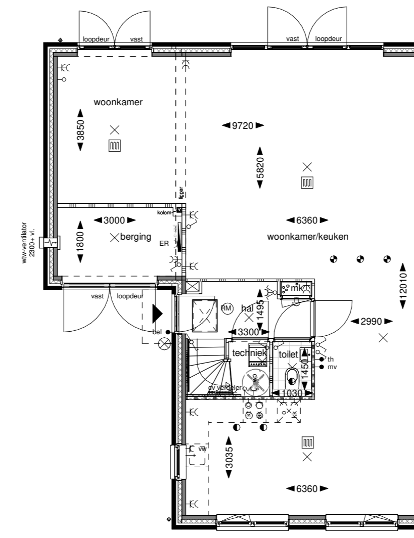
Begane grond
