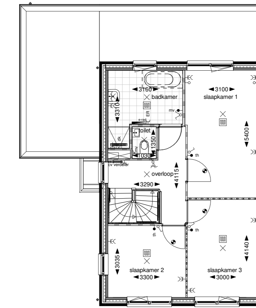
Eerste verdieping
