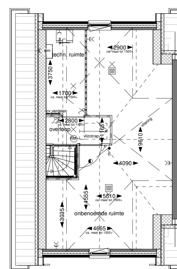
Tweede verdieping
