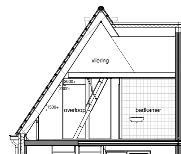
Doorsnede
