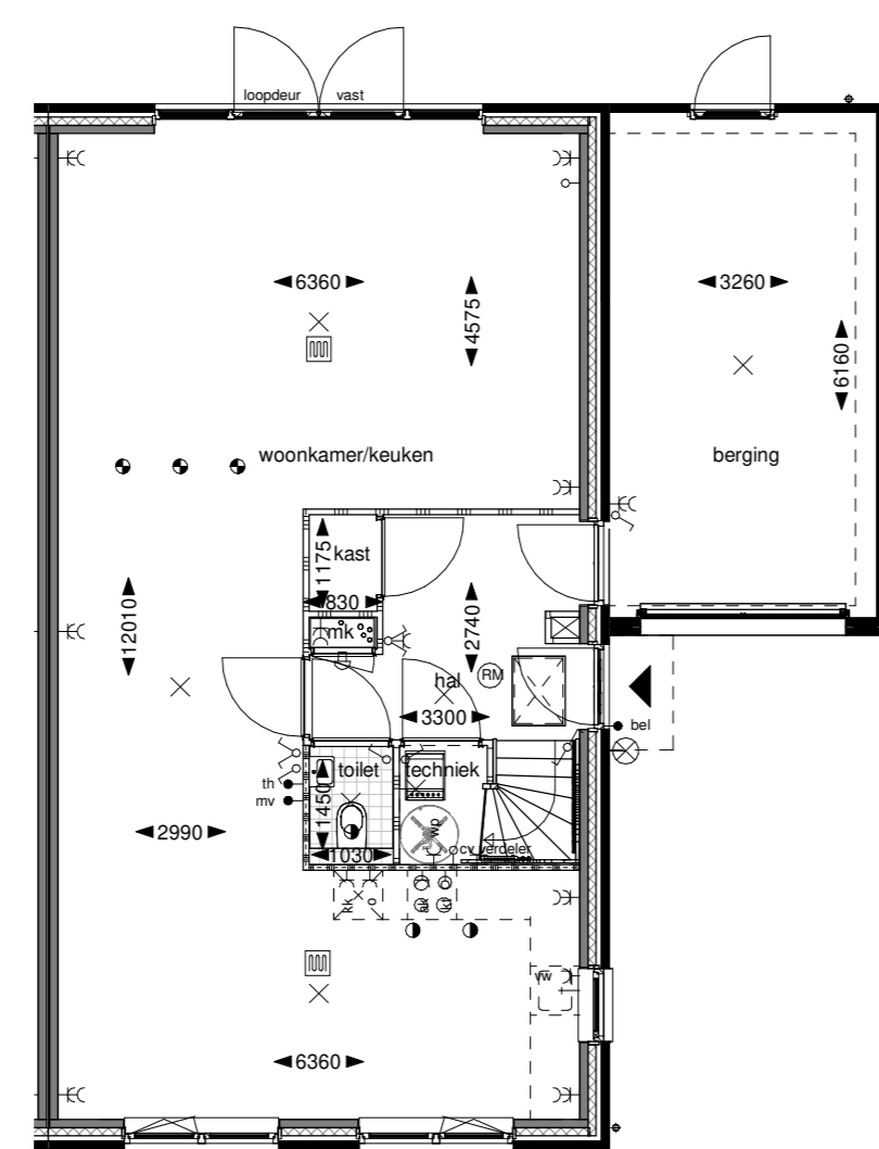
Begane grond
