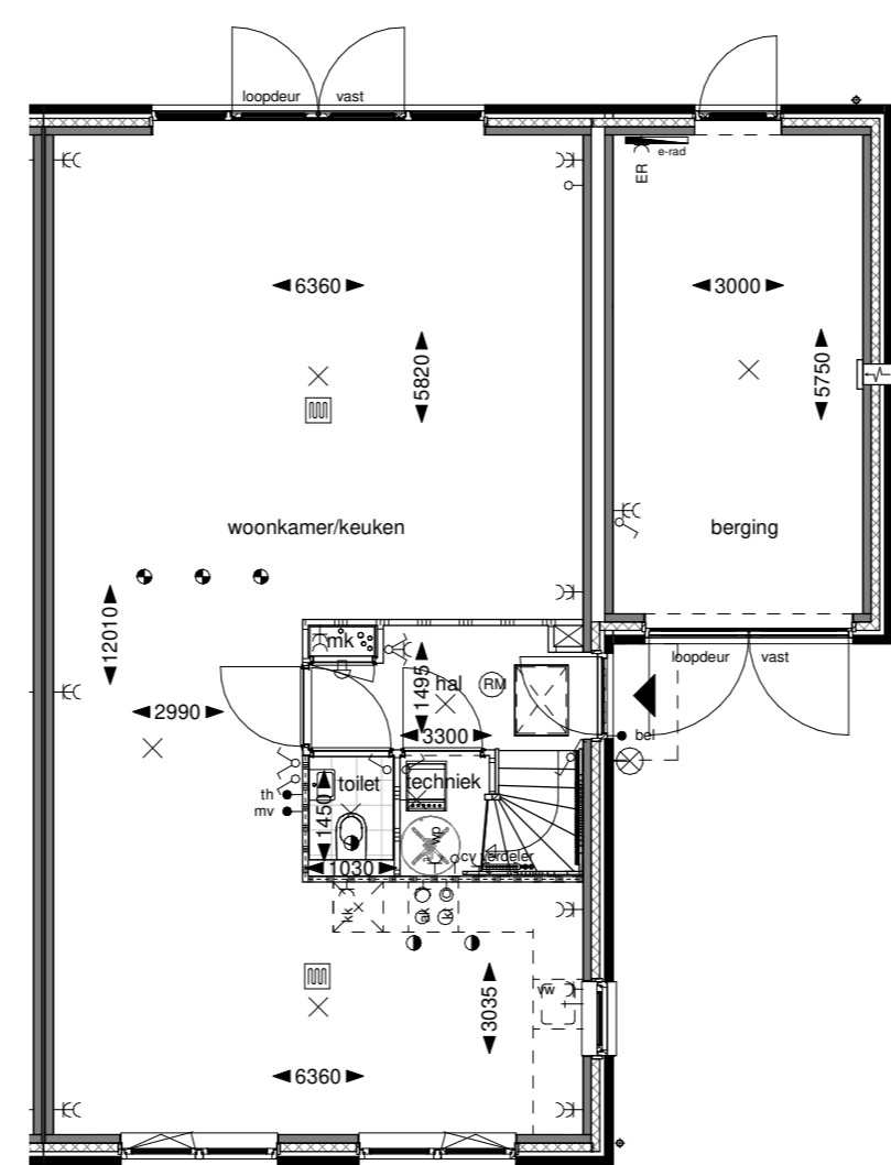
Begane grond
