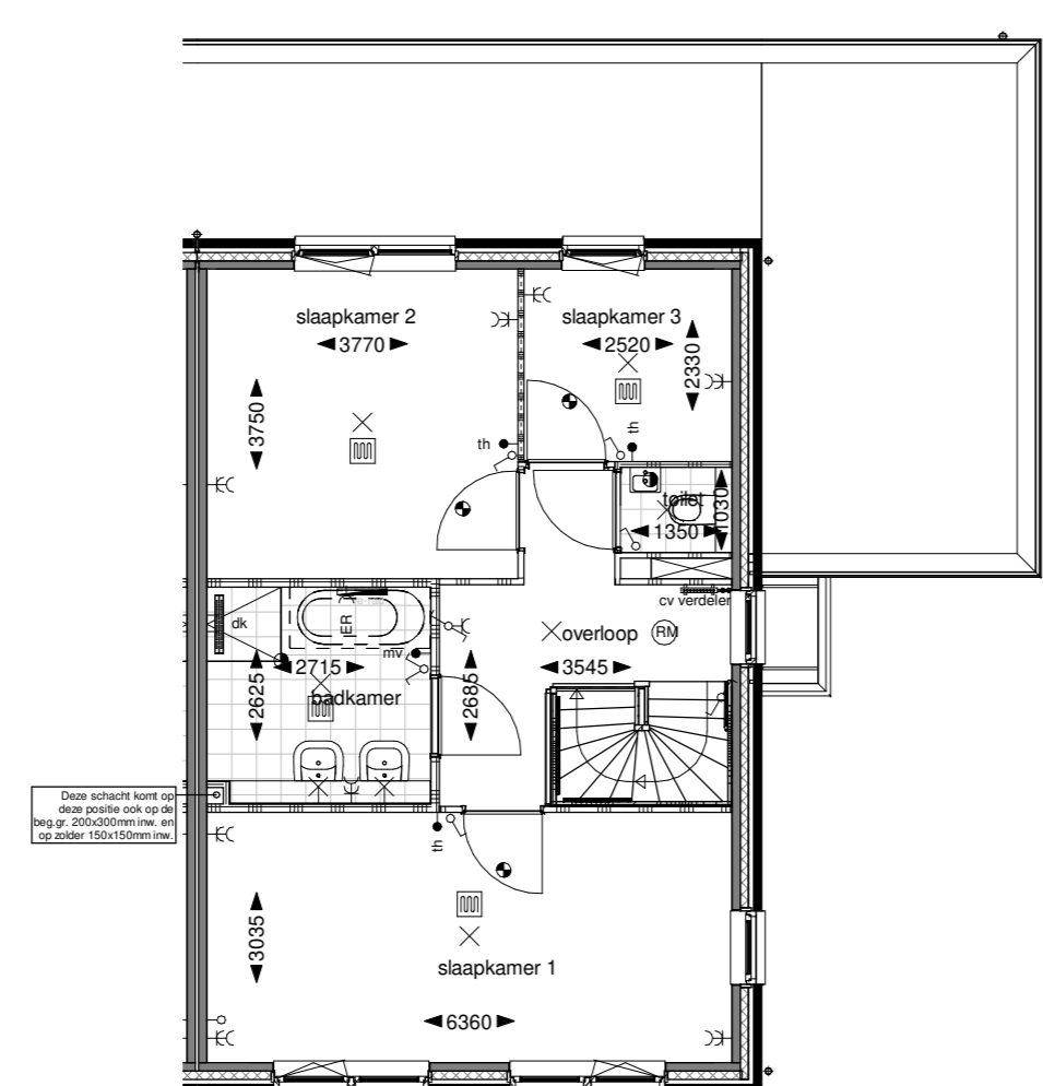
Eerste verdieping
