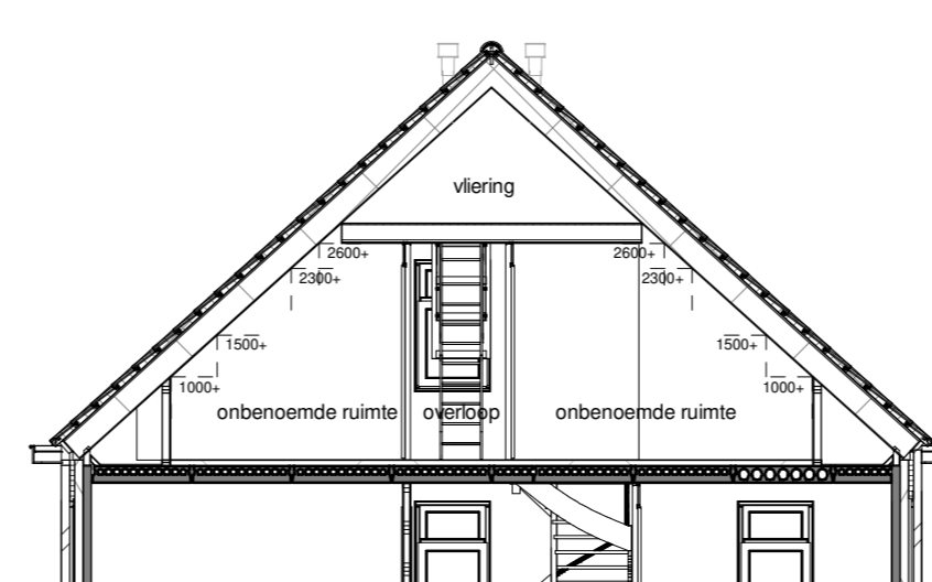
Doorsnede
