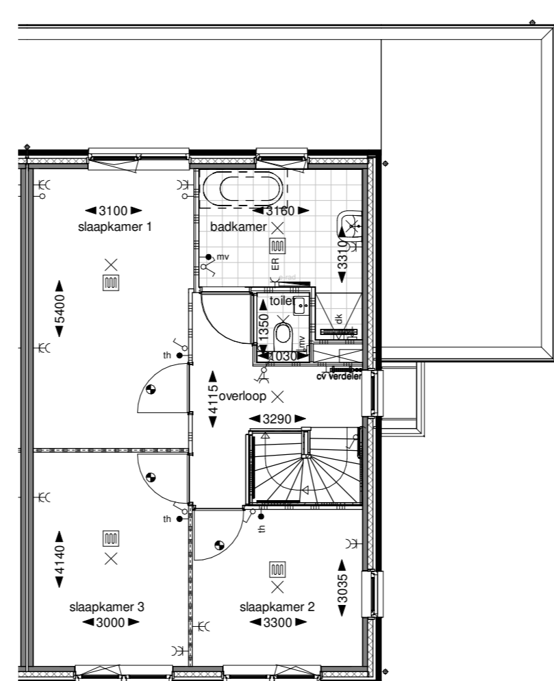
Eerste verdieping
