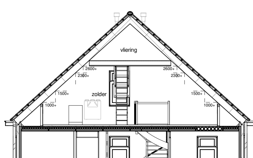
Doorsnede
